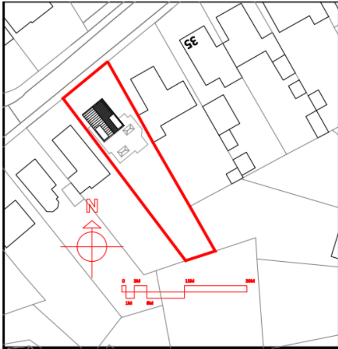
Site plan 1:500
